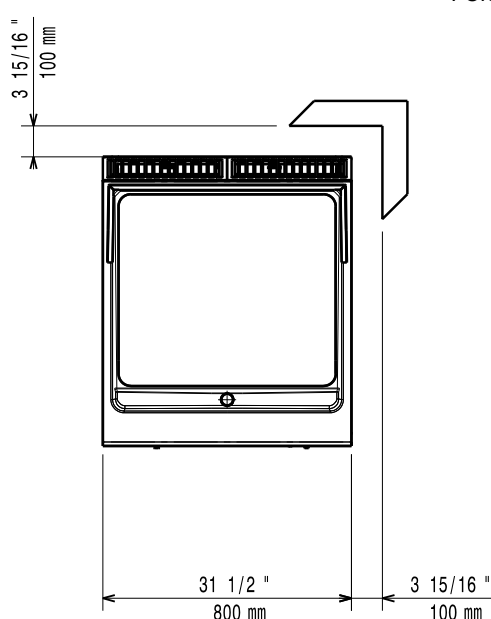
Felülnézet
